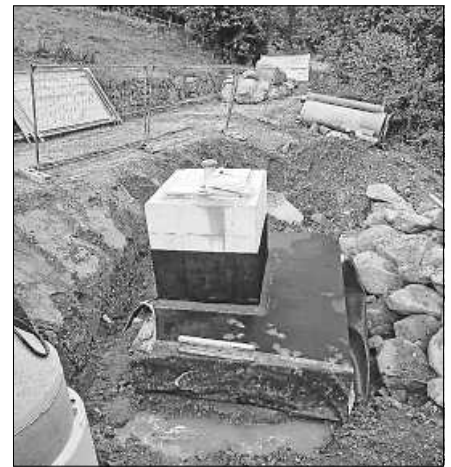
Drosselbauwerk: Dieses dient der Abflussbegrenzung zum Abwassersammler nach Scheuern auf max. 16 l/s.
