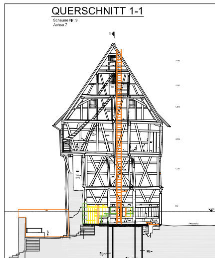
Der Querschnitt zeigt die Position der Leiter in der Scheune. Fotos: B. Säubert
